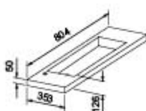
UM 80.120 Раковина 80,4/5/35,3
