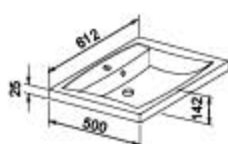
UM 61.110 Раковина 61,2/2,5/50
