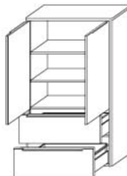
BKG 60.88 Шкаф 69/126,6/36,7
