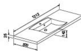
UM 121.110 Раковина 121,2/2,5/50
