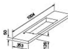
UM 100.120 Раковина 100,4/5/35,3
