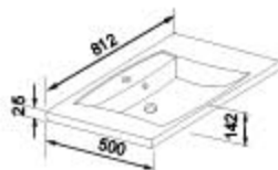
UM 81.110 Раковина 81,2/2,5/50
